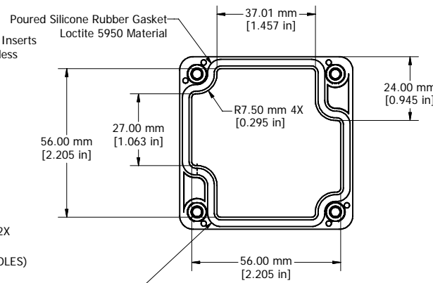
LID - INSIDE
